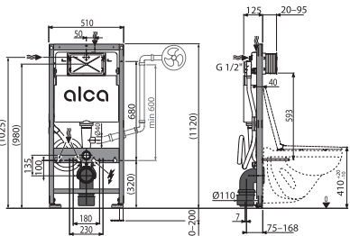
AS120/1120 Sádromodul Скрытая система инсталляции для унитазов с функцией биде
