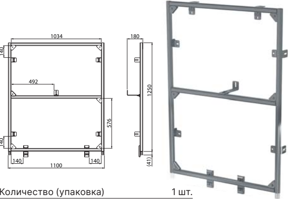
AS101-SET02, AS101-SET02-PR * Системная стена
