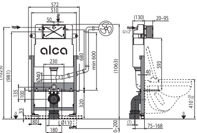
AS101 Sádromodul Скрытая система инсталляции для сухой установки (для гипсокартона)
