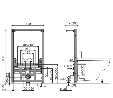
A105/850 Монтажная рама для биде
