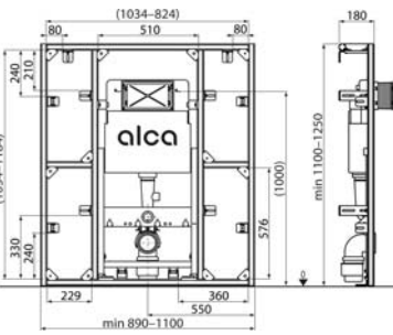
AS101-SET01, AS101-SET01-PR * Системная стена + Скрытая система инсталляции
