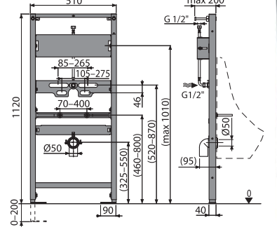
A107S/1120 Монтажная рама для писсуара и сенсорного устройства
