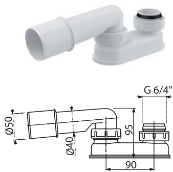
A53-DN50 Гидрозатвор
