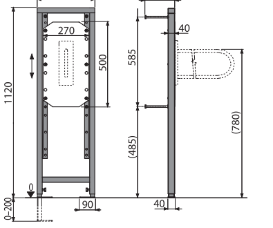
A106/1120 Монтажная рама для поручней
