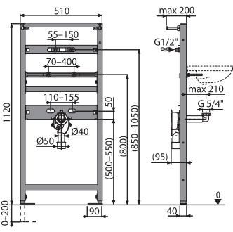
A104AVS/1120 Монтажная рама для умывальника и смесителя со встроенным сифоном
