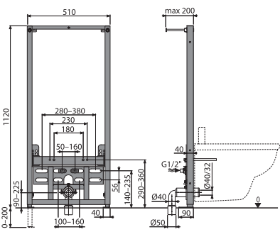
A105/1120 Монтажная рама для биде
