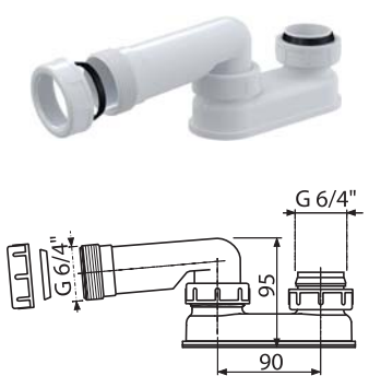
A53-6/4" Гидрозатвор
