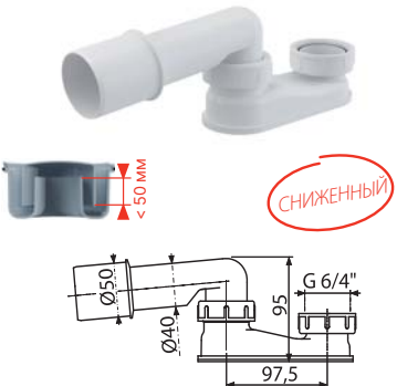
A532-DN50 Сниженный гидрозатвор
