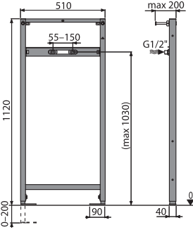
A104B/1120 Монтажная рама для смесителя
